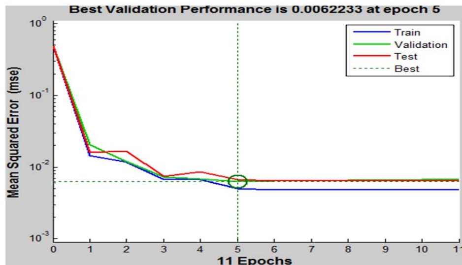
نمودار روند تغییرات خطا در مجموعه‌های آموزش، آزمایش و اعتباردهی کل داده‌ها
